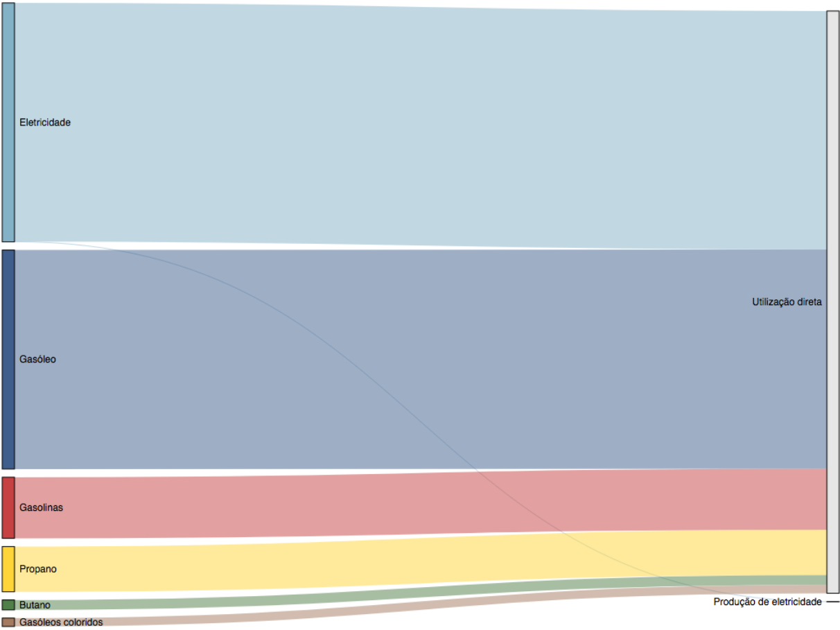
Figura 35: Diagrama de Sankey da utilização de fontes de energia primária no município de Vila de Rei
